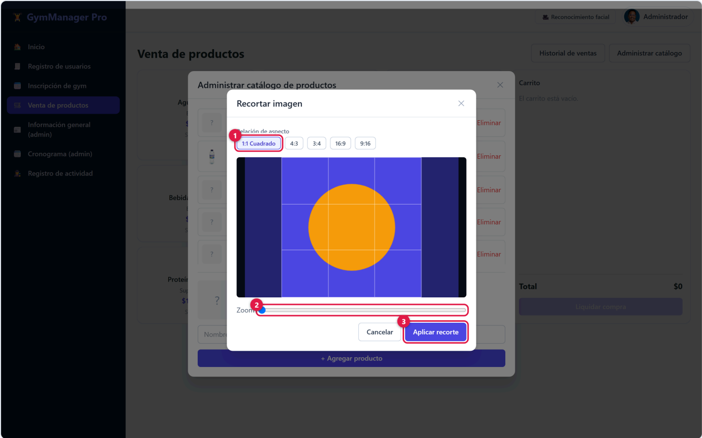
Figura 30. Controles: (1) relaciones de aspecto disponibles, (2) control de zoom, (3) Aplicar recorte.
