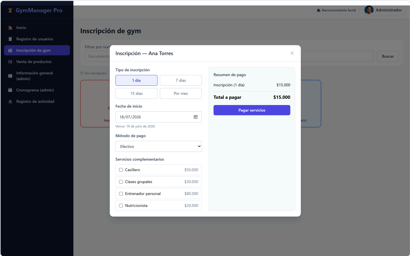
Figura 16. Ventana de inscripción: duración, fecha de inicio, método de pago, servicios complementarios y resumen de pago.
